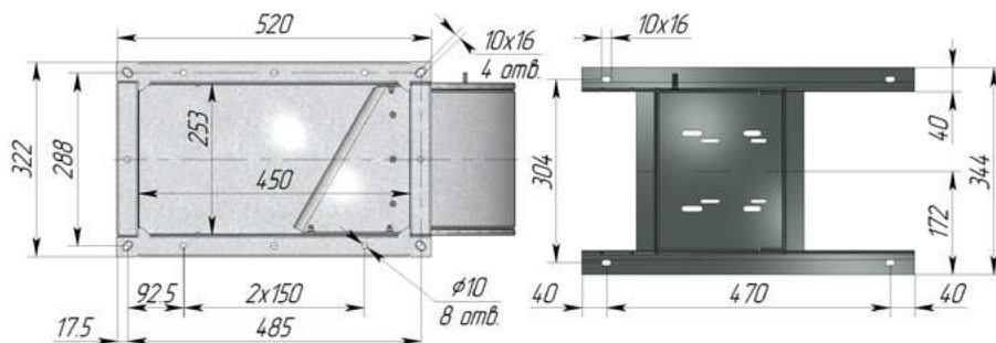
Выходной фланец
