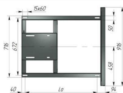
Опорная рама
