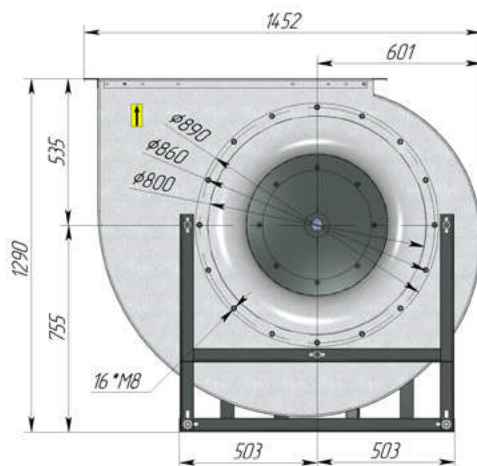
Выходной фланец
