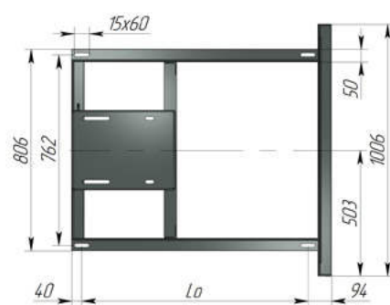
Опорная рама
