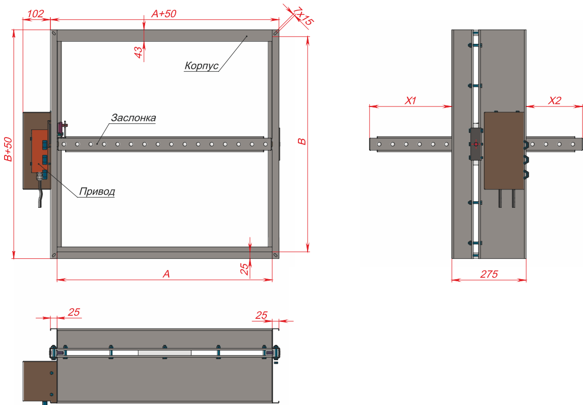
Клапан mcr FID-120-K1-A×B прямоугольного сечения с электромеханическим приводом
