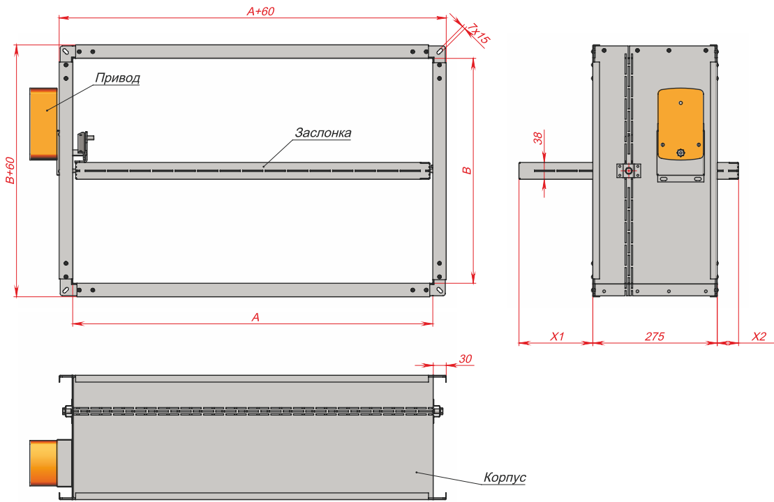
Клапан mcr FID-60/90-K1-A×B прямоугольного сечения с электромеханическим приводом
