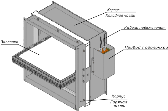
mcr FID-30-K1 двойного действия
