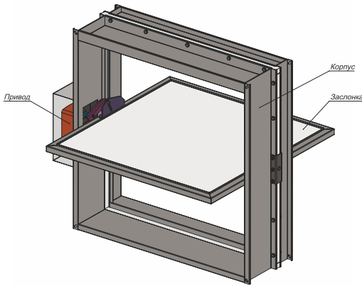
mcr FID-30-K1 двойного действия
